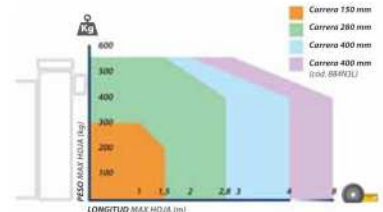
La estructura, la forma (con paneles cerrada), la altura de la puerta y las condiciones climáticas pueden reducir los valores mostrados. Compruebe siempre la integridad de la estructura de la puerta
