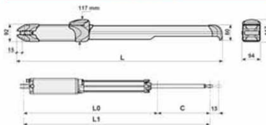
La estructura, la forma (con paneles cerrada), la altura de la puerta y las condiciones climáticas pueden reducir los valores mostrados. Compruebe siempre la integridad de la estructura de la puerta
